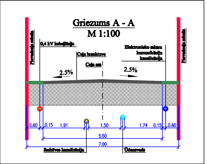
Piebraucamā ceļa šķēršprofils, M 1:100
